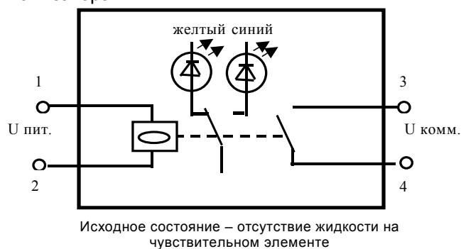
Рисунок 1 – Блок-схема сигнализатора
