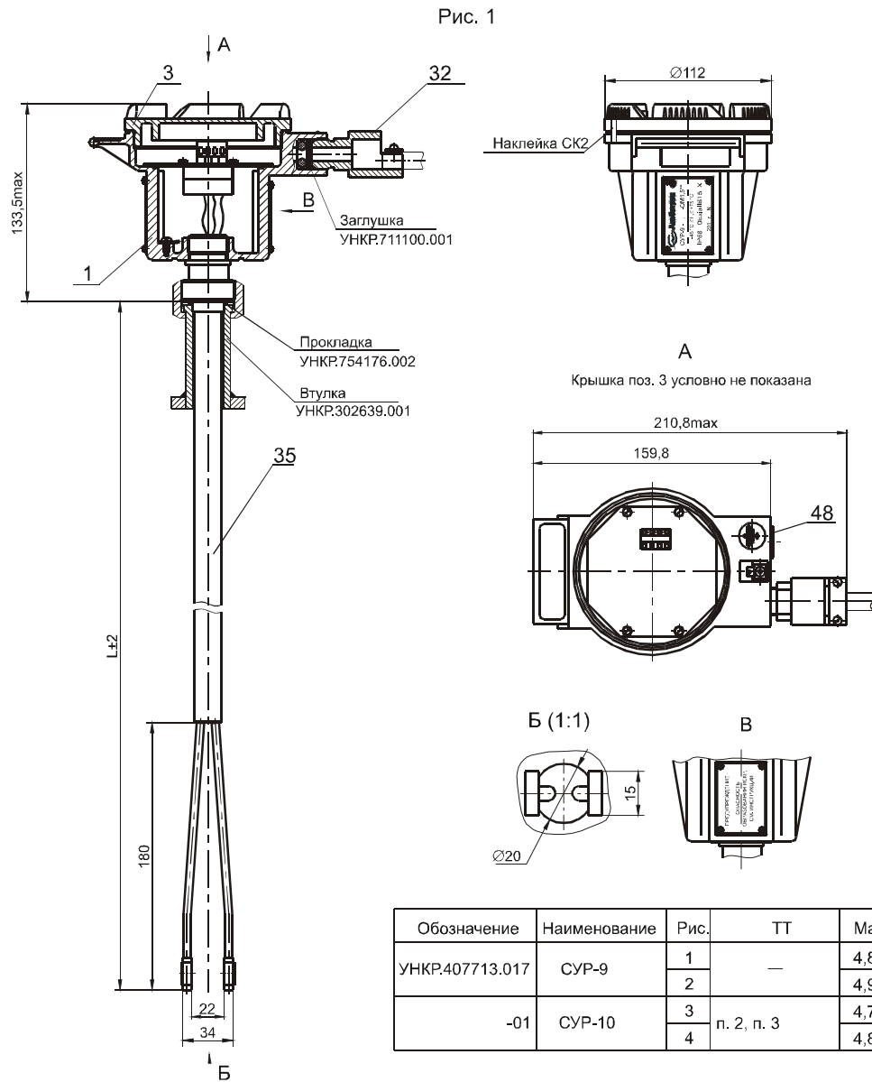
Рисунок В.1 - Габаритные и установочные размеры сигнализатора СУР-9, СУР-10 (лист 1)
