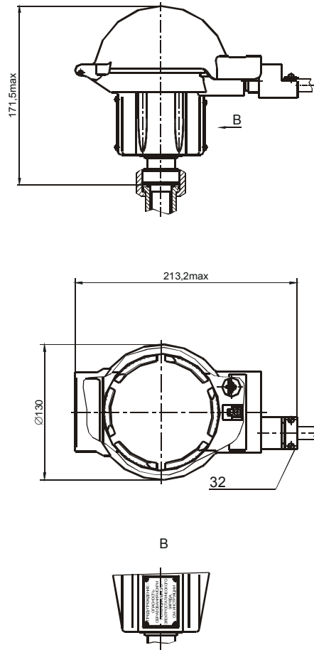
Рисунок В.2 - Габаритные и установочные размеры сигнализатора СУР-9, СУР-10 (лист 2)
