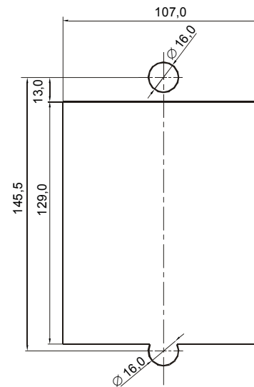
Рекомендуемое посадочное место для установки ПВС8
