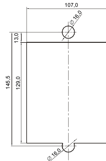
Рекомендуемое посадочное место для установки ПВС7
