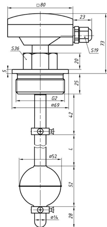
Рисунок А.1 - Габаритные размеры
