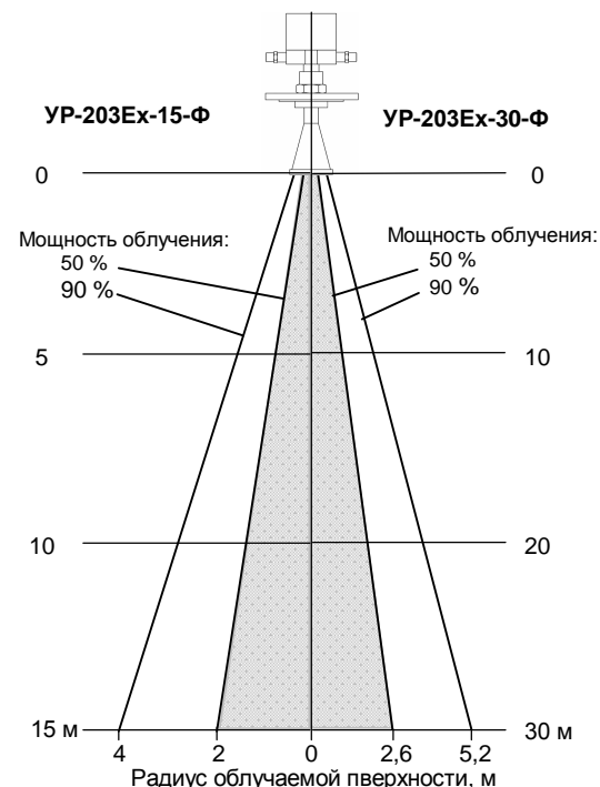
Рис. 2 – Диаграмма направленности антенны
