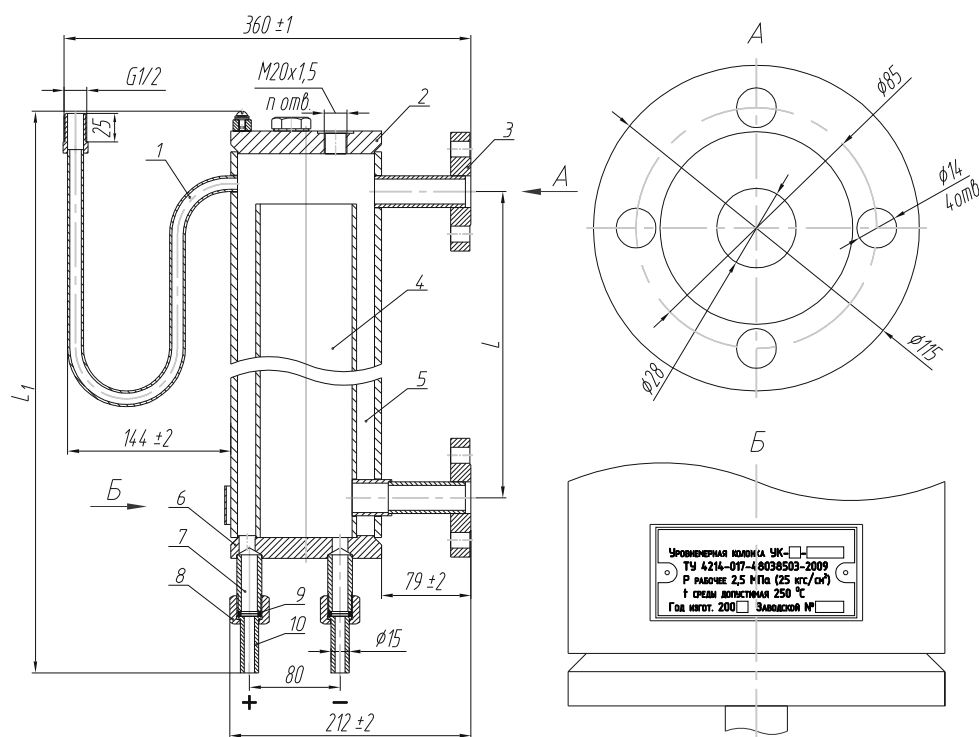
Рисунок 1 - Устройство колонки
