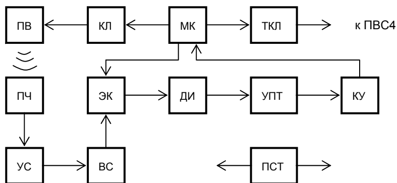
Рисунок 1 – Структурная схема датчика
