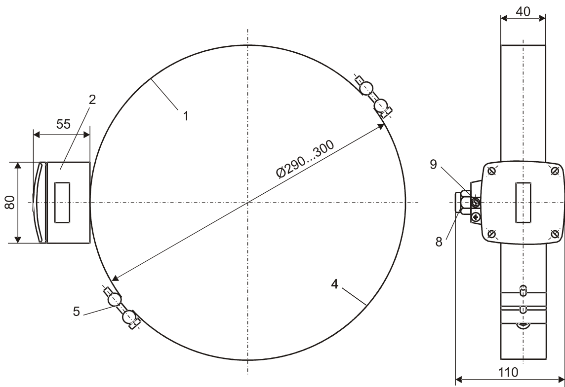
Рисунок 10 - Датчики исполнения ЕС 86ХИ
