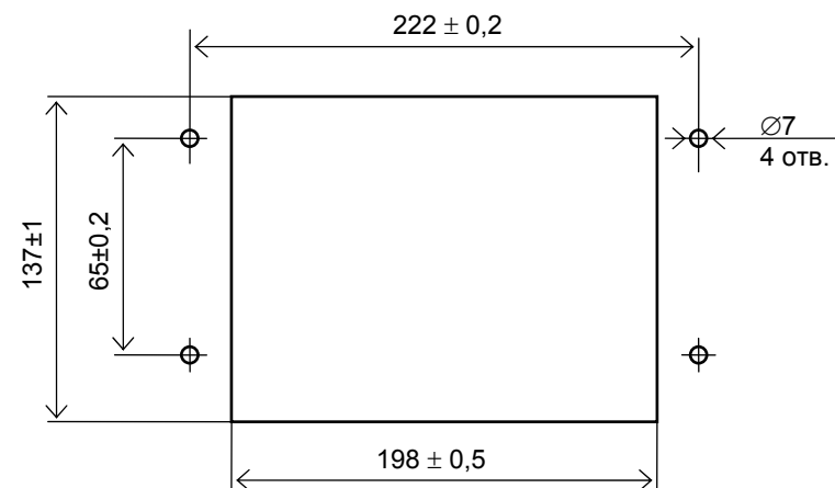
Рисунок 7 – Рекомендуемое посадочное место для установки прибора
