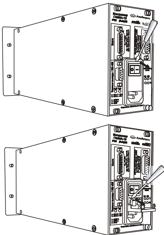
Рисунок 5 – Замена вставок плавких на задней стороне прибора 13 ТЕХНИЧЕСКОЕ ОБСЛУЖИВАНИЕ И ПОВЕРКА ПРИБОРА
